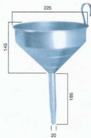
Código 613 Modelo Médio para trator
