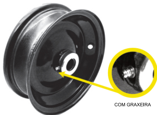
ARO METÁLICO 8" POL - C/ GRAXEIRA - PRETO
