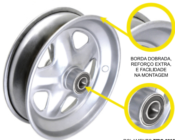
ROLAMENTO TIPO 6205
